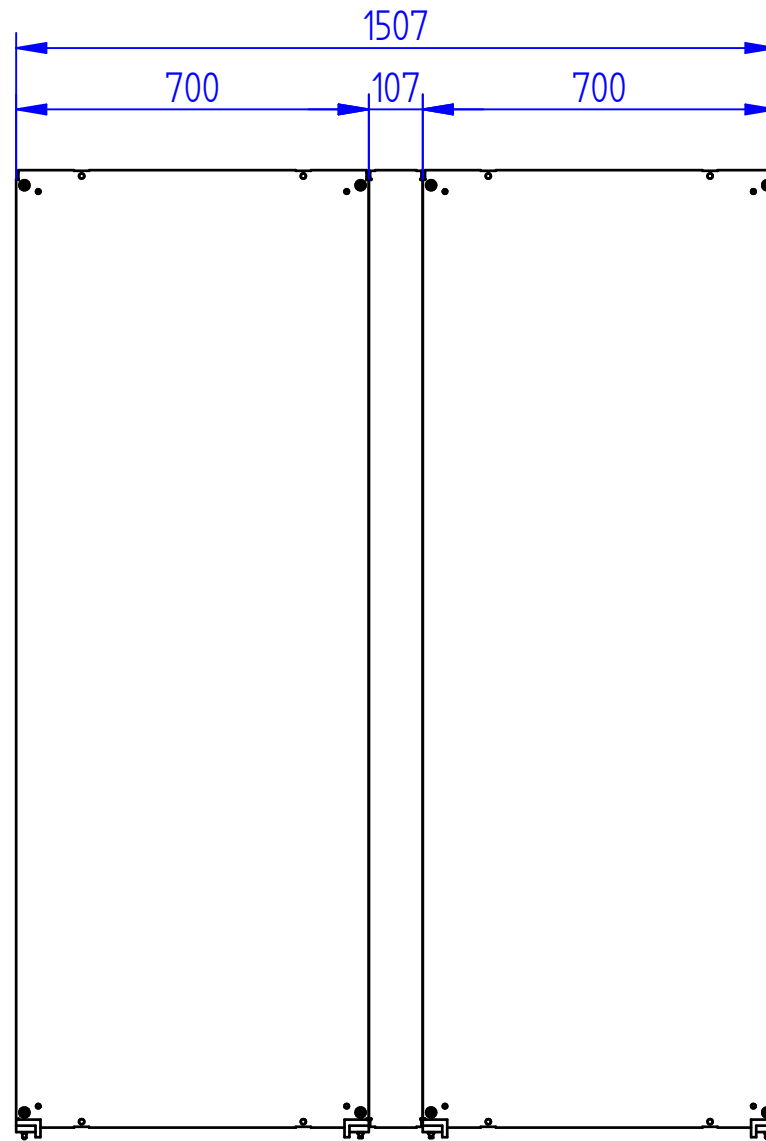
*PLACA DE MONTAJE PARA MÓDULOS DE L.1600
