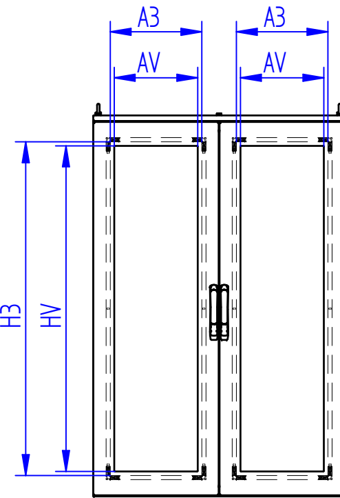
VERSIÓN CON MONTANTE CENTRAL EXTRAÍBLE
